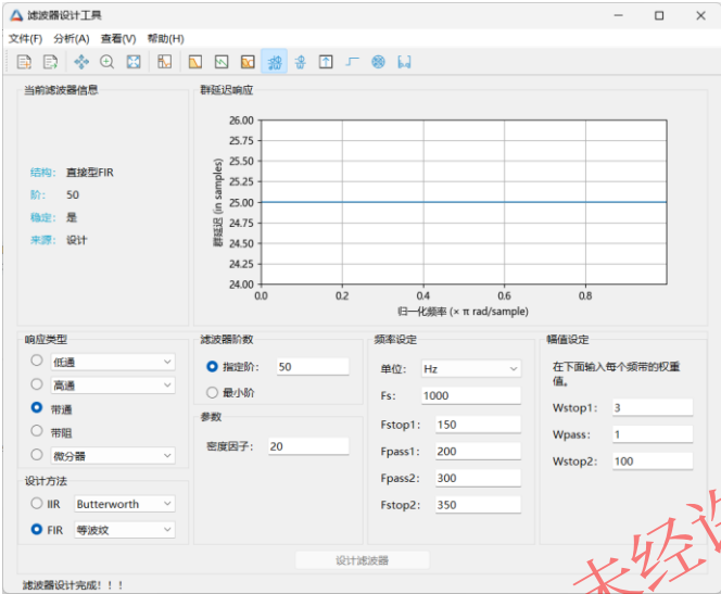
群延迟响应
