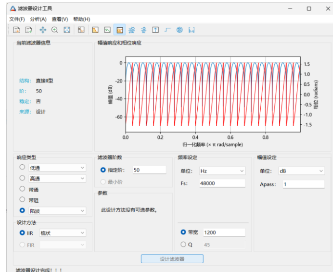
示例6: 梳状滤波器
