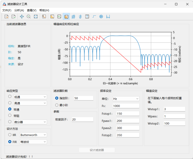
幅值响应和相位响应
